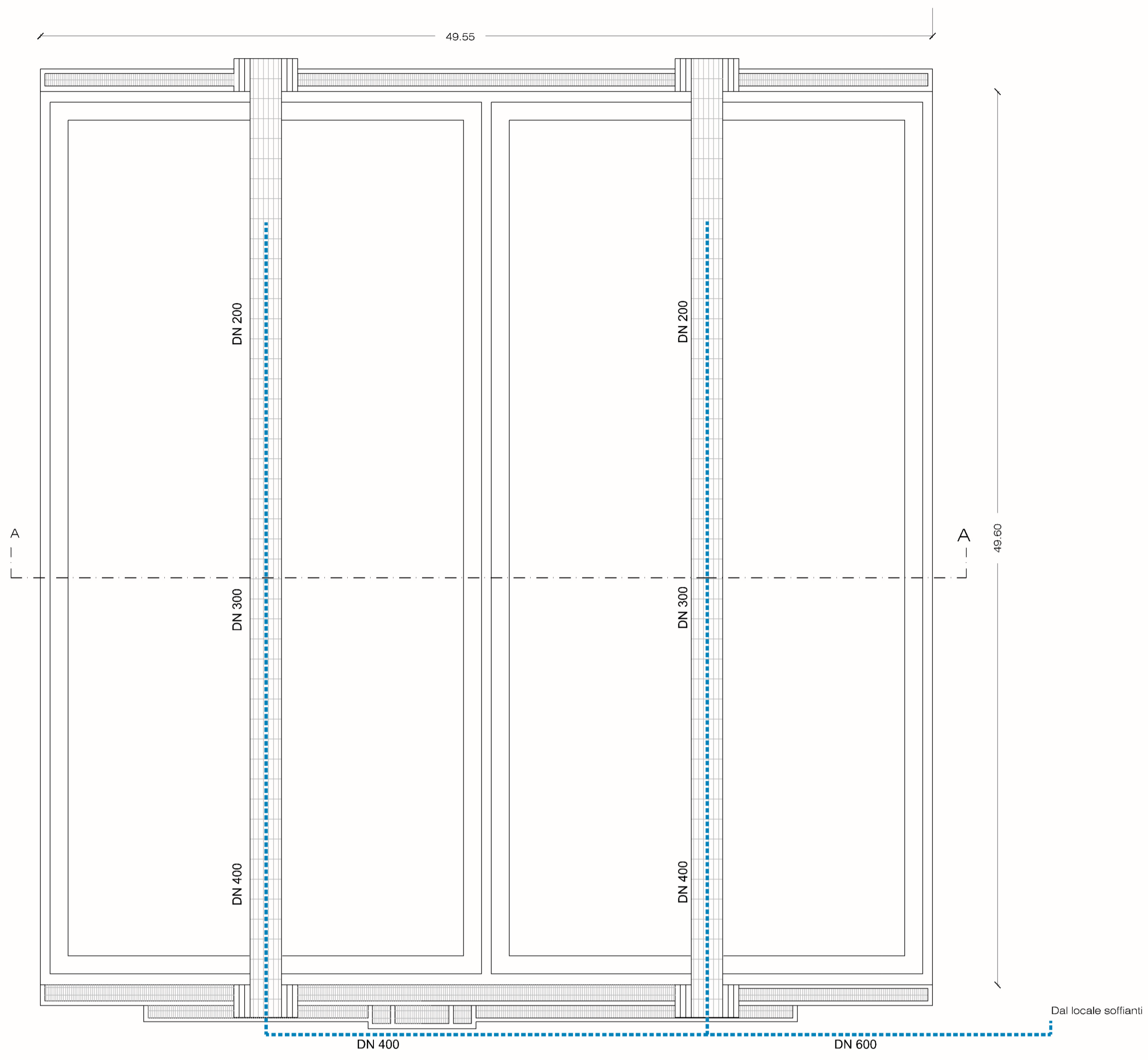
PIANTA
